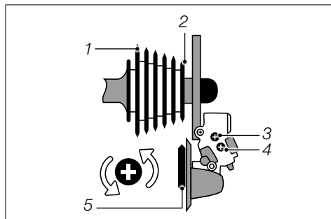
Abb.: Darstellung eines Schaltwerks (exemplarisch)
