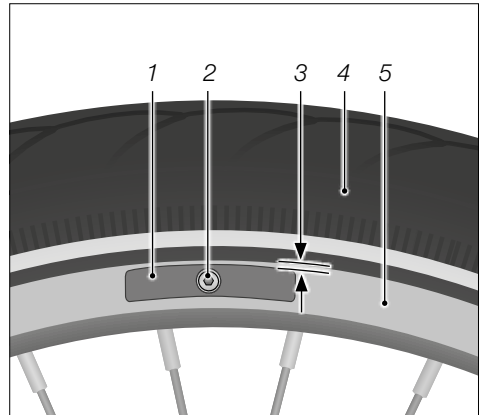
Abb.: Ausrichtung Bremsstufe (exemplarisch)
