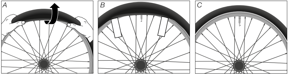
Abb.: Draht- oder Faltreifen montieren (exemplarisch)
