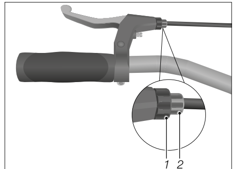
Abb.: Position Kontermutter und Rändelschraube (exemplarisch)
