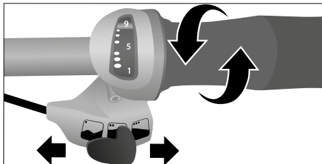
Abb.: Kombiniertes Drehgriff- und Schalthebelschalter Dual Drive (exemplarisch)
