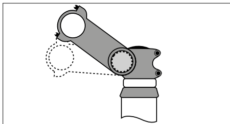
Abb.: Neigungsverstellung (exemplarisch)
